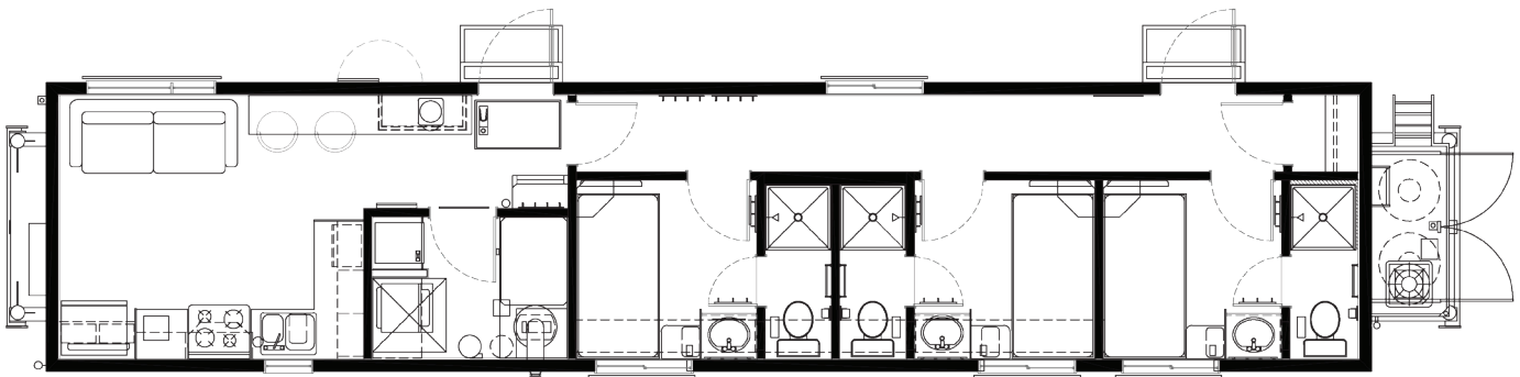
1 A-1 3 PERSON STAFF QUARTERS SCALE: N.T.S.
